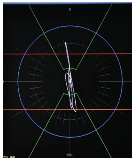
Display polar da tela EC mostrando o sinal de um furo passante num tubo de cobre.
