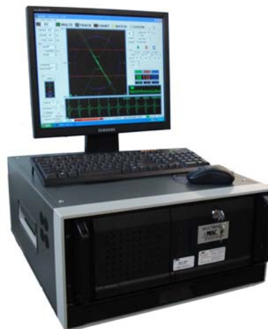
Menú Principal del MultiMac mostrando simultáneamente los gráficos polar y linear de un canal de prueba incluyendo todos los parámetros de ajuste. La pantalla Multi (pagina 3) puede mostrar los gráficos polar y linear de hasta 8 canales.
