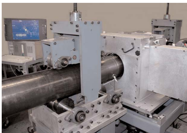
Cabeçote rotativo Rotomac ® Modelo 750 para inspecionar tubos ou barras com diâmetros externos até 7 1/2" (190,5 mm), para operar em linha com uma endireitadeira ou num sistema fora de linha. O cabeçote rotativo é normalmente montado sobre uma mesa de elevação com ajuste lateral e de altura e numa mesa central de teste da MAC.
