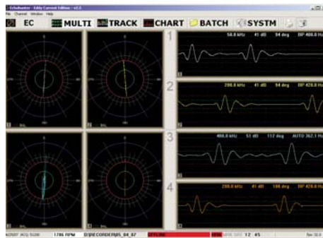
Tela Multi do MultiMac SM mostrando simultaneamente os displays polar e linear de quatro canais de teste, assim como os respectivos limiares de alarme. A tela Multi pode mostrar os displays polar e linear de até 4 canais.
