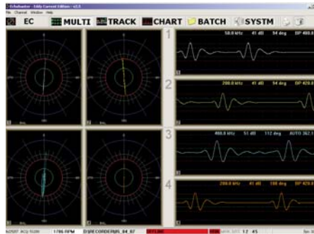
MultiMac 多屏幕同时显示4条信道的极性 & 线性画面。最多8条通道，具有全部阈值，均可同时显示。
