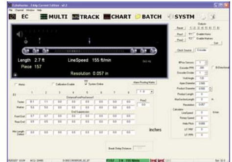
MultiMac端抑制屏幕用于为端传感器输入数据。
