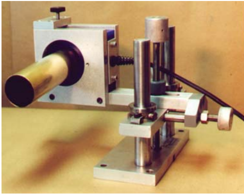
30系列环绕检测线圈平台
