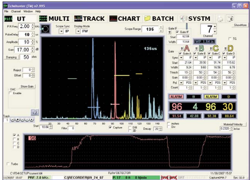
Echomac FD4 – UT超声波检测仪的设置显示
