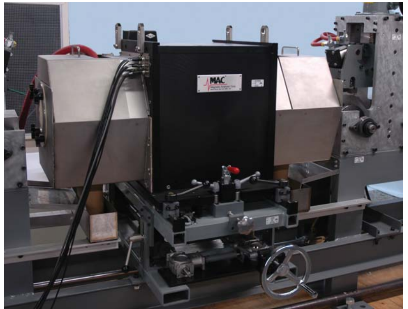
MAC Echomac 七信道超声波旋转装置安装在较高的平台上，用于检测4英寸（101.6毫米）直径的材料。旋转式传感器置于黑匣子内，加压水耦合剂也装在里面。
